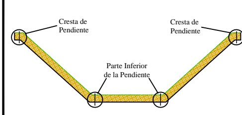
Figura G - Sujeción de Puntos Críticos
